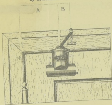
Fig. 1. Puerta derecha con resorte accionando a la derecha.
