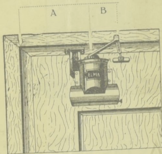
Fig. 3. Puerta izquierda para afuera con resorte accionando a la derecha.
